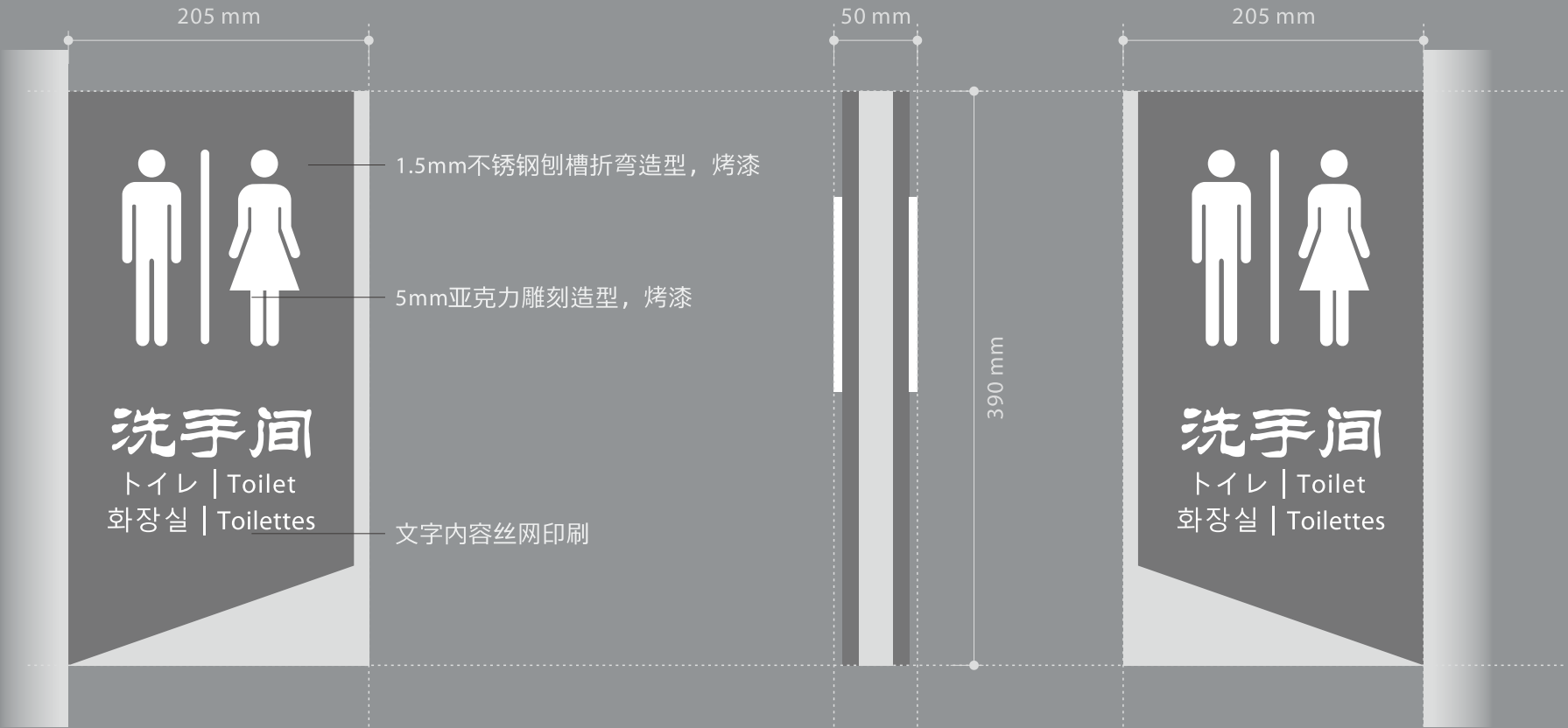
正视图/FRONT
