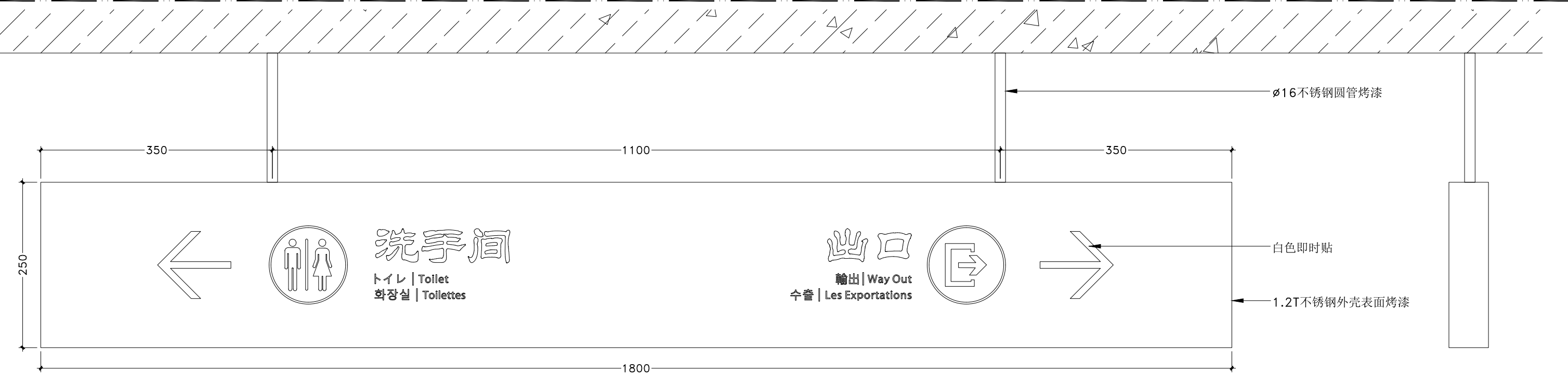
正视图
