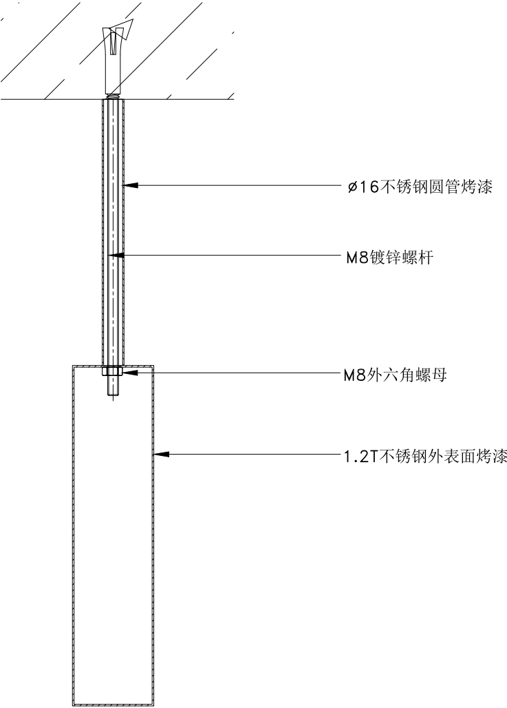
侧剖图
