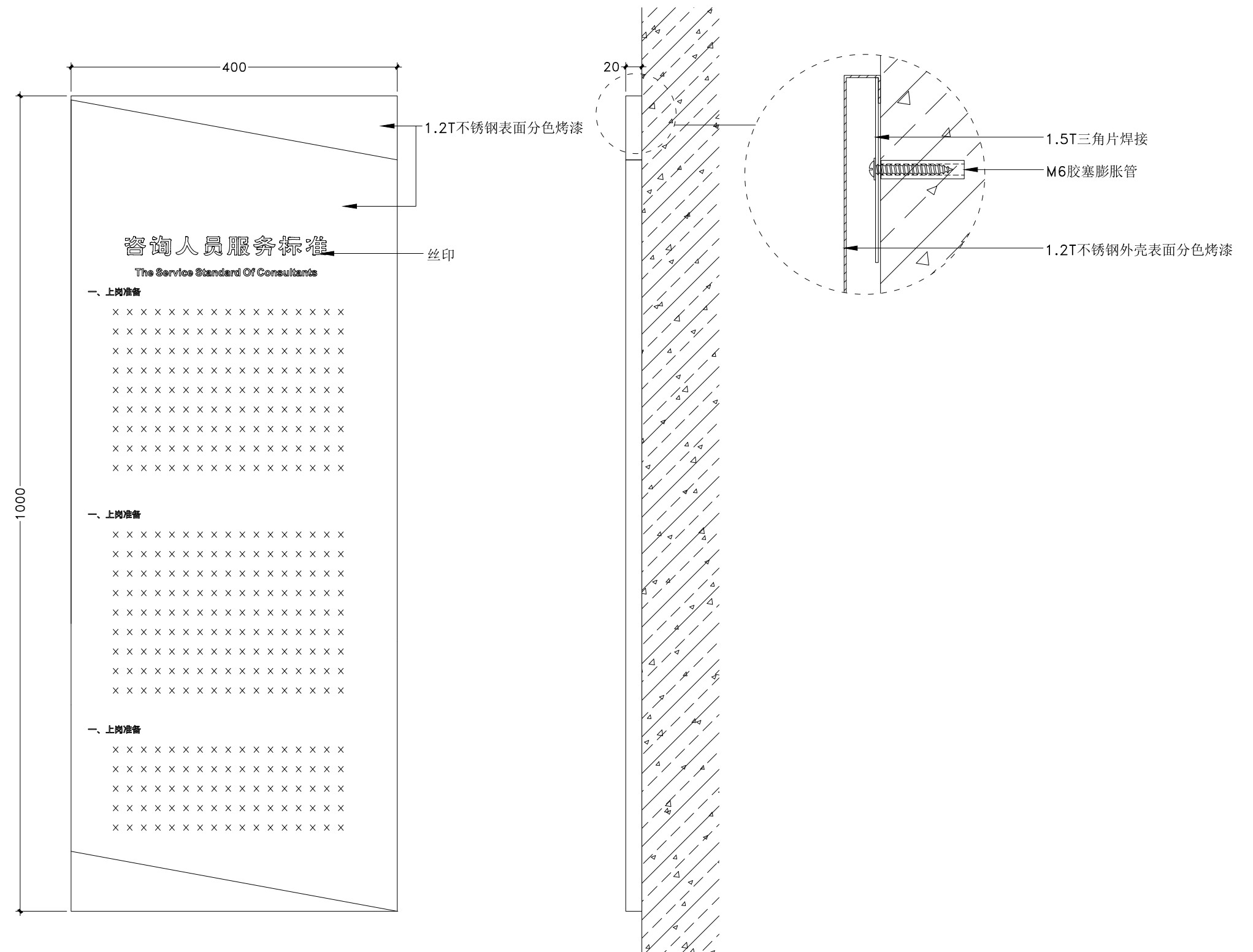
正视图
